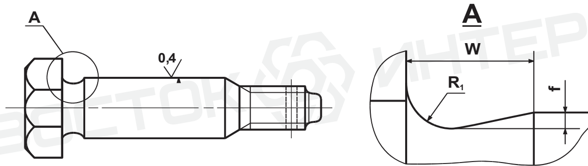
Исполнение 2 (Исполнение 2а - без отверстия под шплинт)
